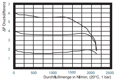
Filterdruckminderer Baugröße 1
