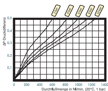
Nebelöler Baugröße 1
