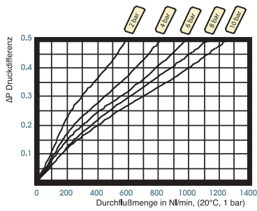
Filterwasserabscheider Baugröße 1
