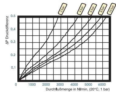
Baugröße 3
