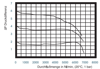
Baugröße 3
