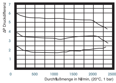
Druckminderer Baugröße 1
