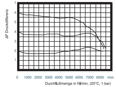
Baugröße 3
