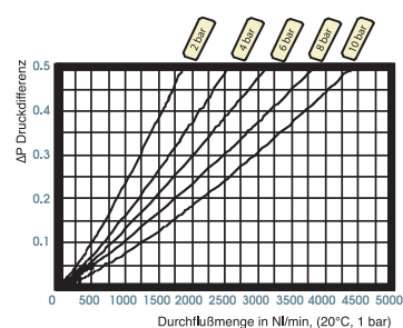
Baugröße 2
